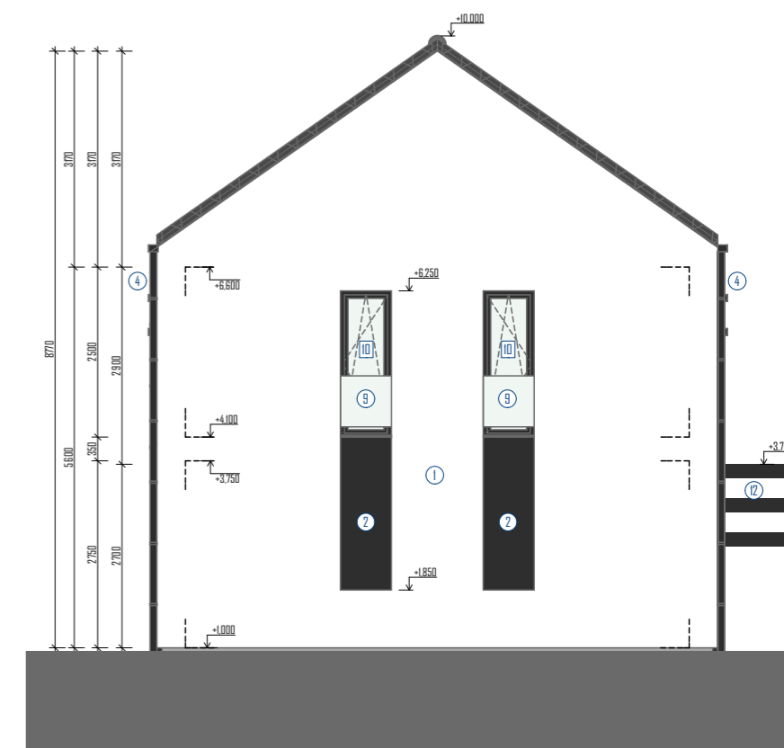
SO-103_POHLED JIŽNÍ
