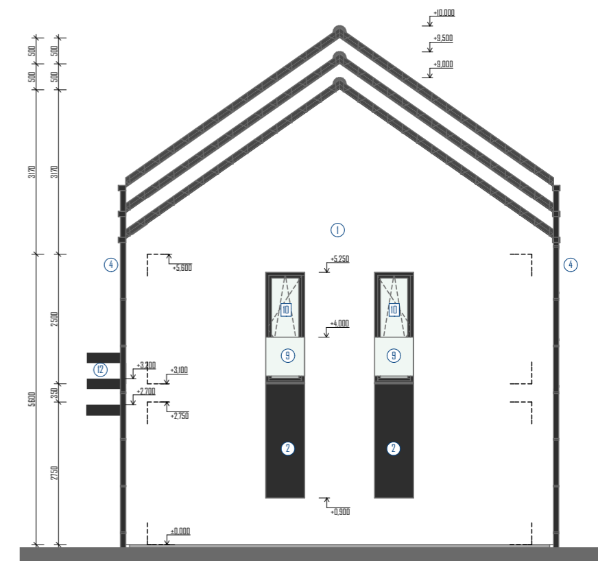
SO-103_POHLED SEVERNÍ
